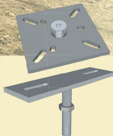
un éco-système d'accessoires pour créer tous types de fondations
